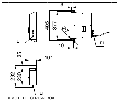
CONTROLLER - 1PC
